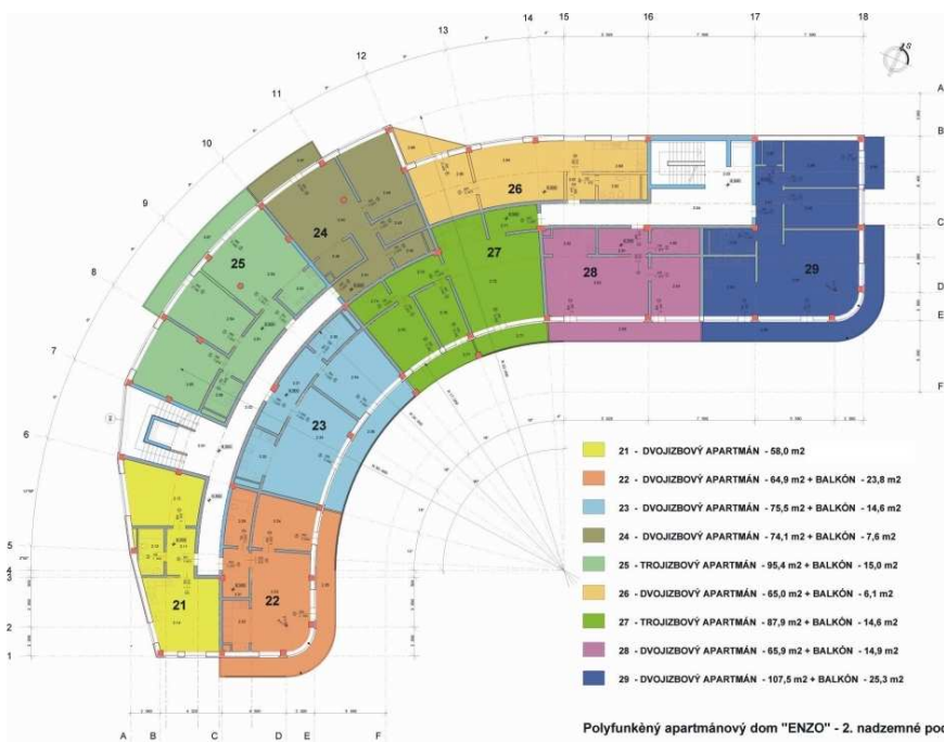
Polyfunkčný apartmánový dom "ENZO" - 2. nadzemné podlažie
